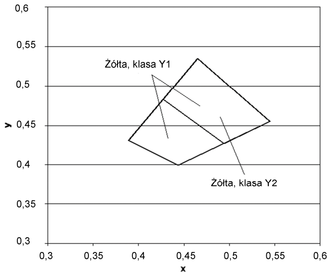
Rys.2. Współrzędne chromatycyjnosc x,y dla barwy zoltej oznakowania
