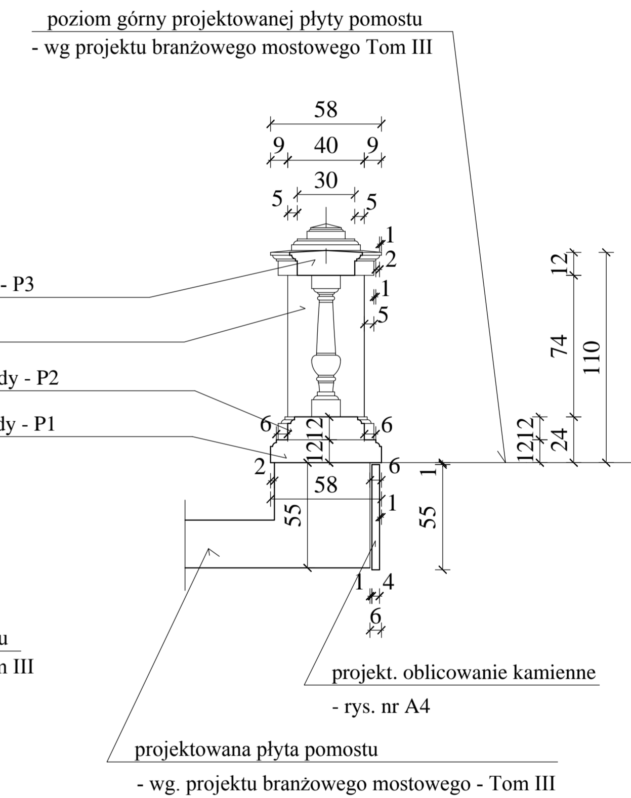
PRZEKRÓJ A - A 1 : 20
