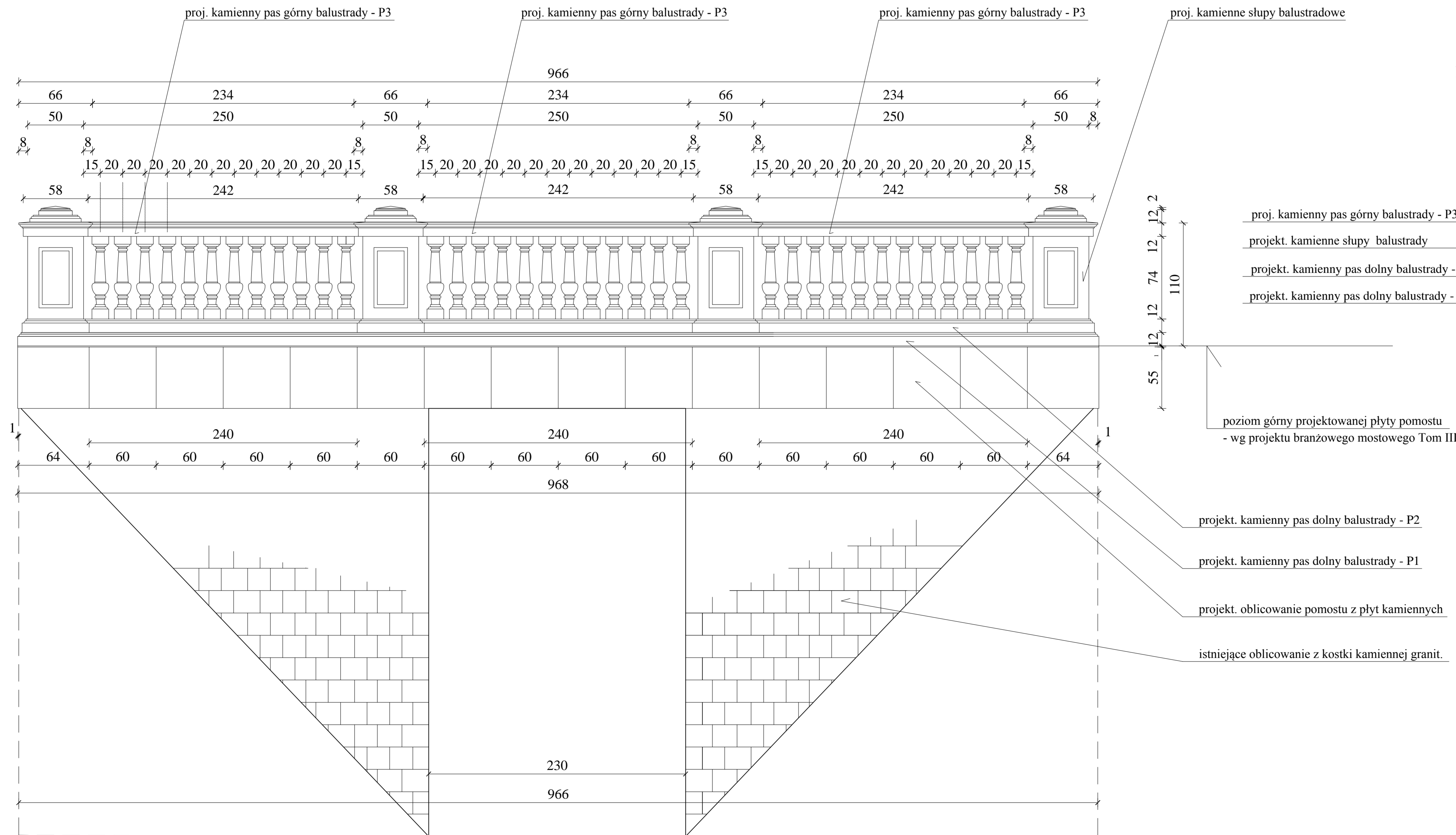
WIDOK MOSTU Z BOKU 1 : 20
