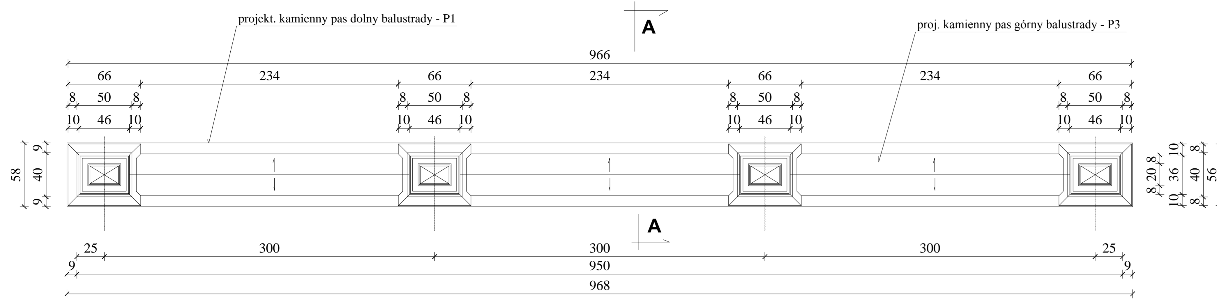
WIDOK BALUSTRADY Z GÓRY 1 : 20
